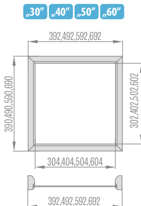
Supralumini de colț ale tocului fix
