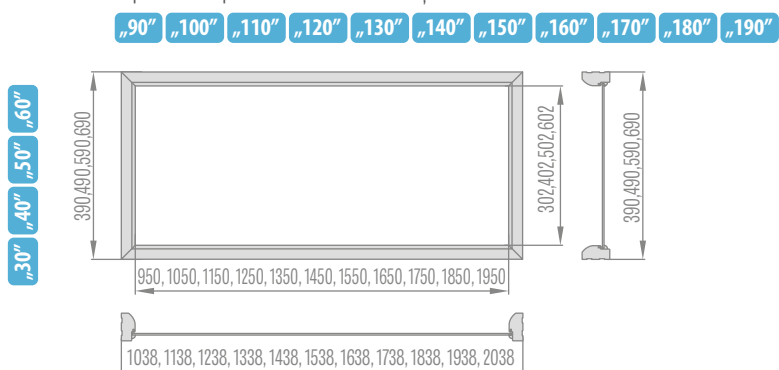
Supralumini superioare ale tocului fix la o ușă cu două canaturi
