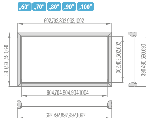
Supralumini superioare ale tocului fix la o ușă cu un canat
